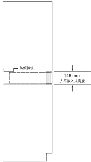
侧视图
