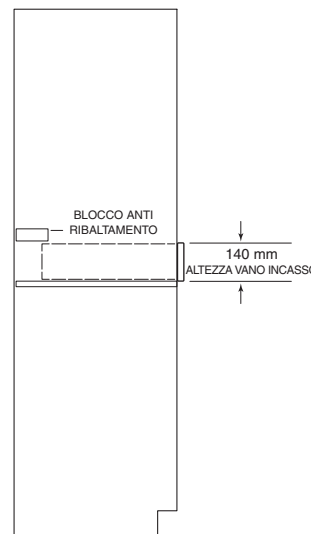
VISTA LATERALE
