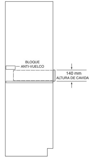
VISTA LATERAL
